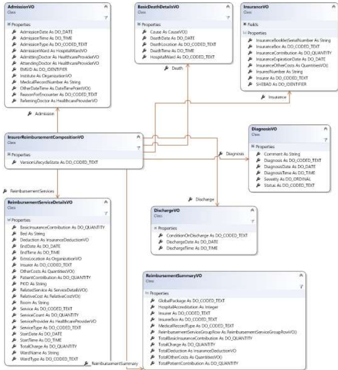
شکل ۴- کلاس InsurerReimbursementCompositionVO
