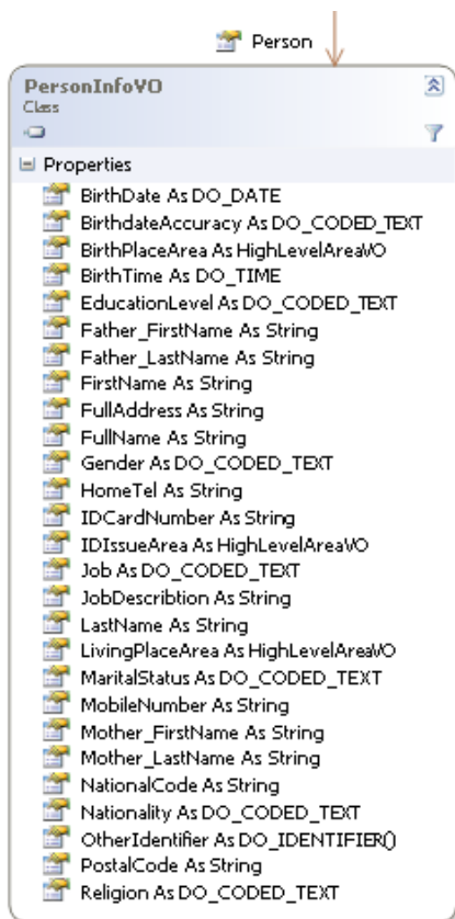
شکل ۶- کلاس PersonInfoVO و اجزای آن
