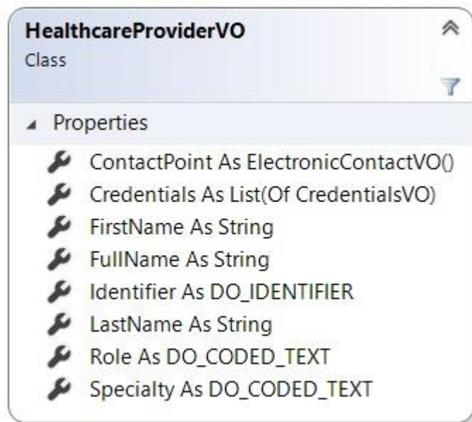
شکل ۴ - کلاس HealthcareProviderVO
