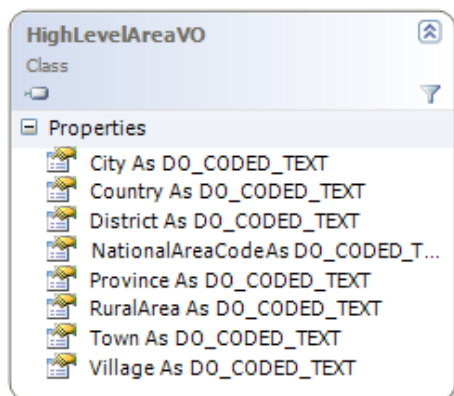
شکل ۸ - کلاس HighLevelAreaVO
