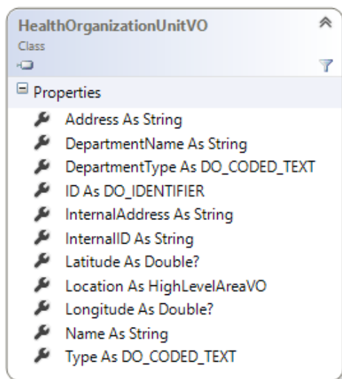
شکل ۷ - کلاس HealthOrganizationUnitVO
