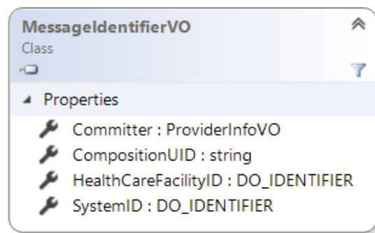
شکل ۳ - کلاس MessageIdentifierVO
