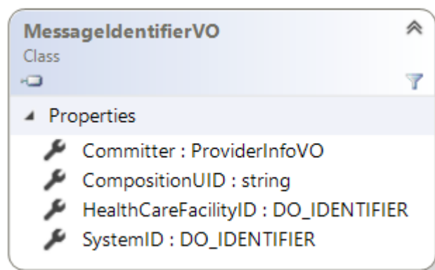
شکل ۲ - کلاس MessageIdentifierVO
