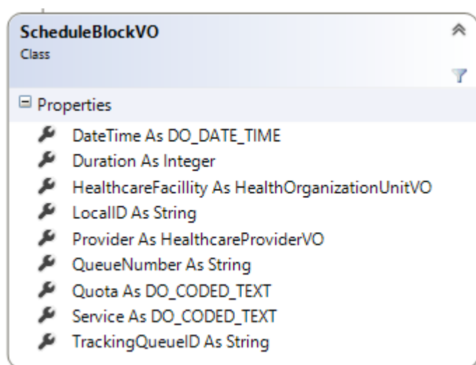
شکل ۹- کلاس ScheduleBlockVO
